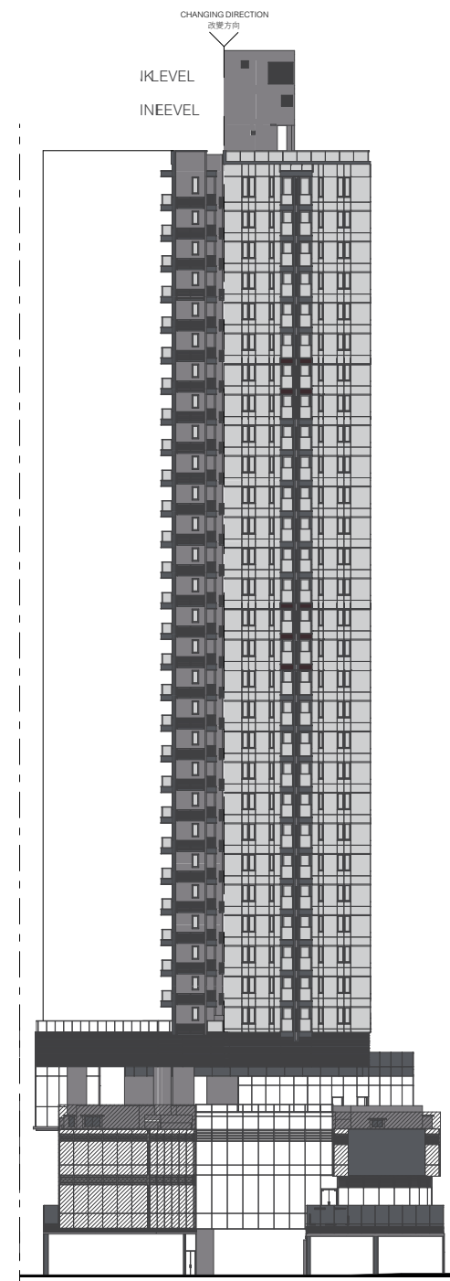
Elevation Plan B 立面圖 B
