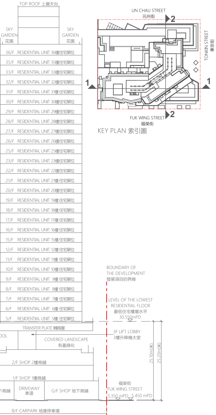
CROSS-SECTION PLAN 2 橫截面圖 2
